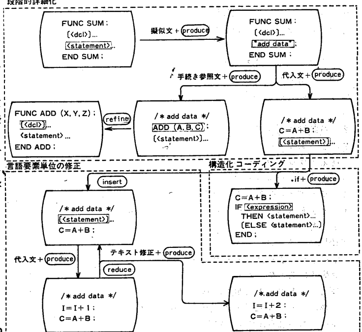
図2 PARSEを用いたプログラム編集例
