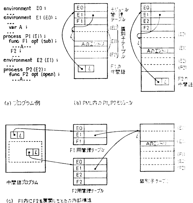
図5 手続きのインライン展開のメカニズム
